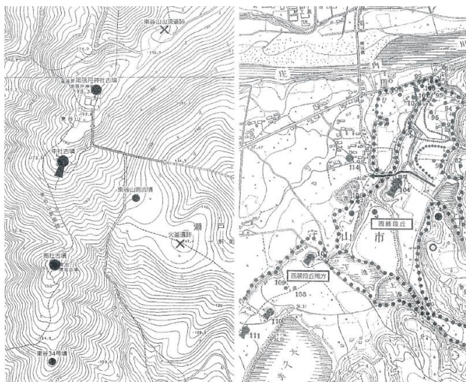
図2 東谷山山峰の墓域図 (1/5,000)
